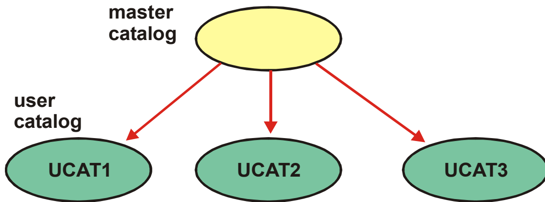
Catalog hierarchy
